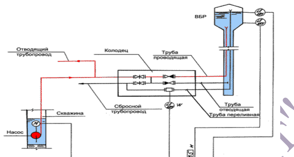
Рис.. Схема водоснабжения населенного пункта при заборе воды из подземных источников.
